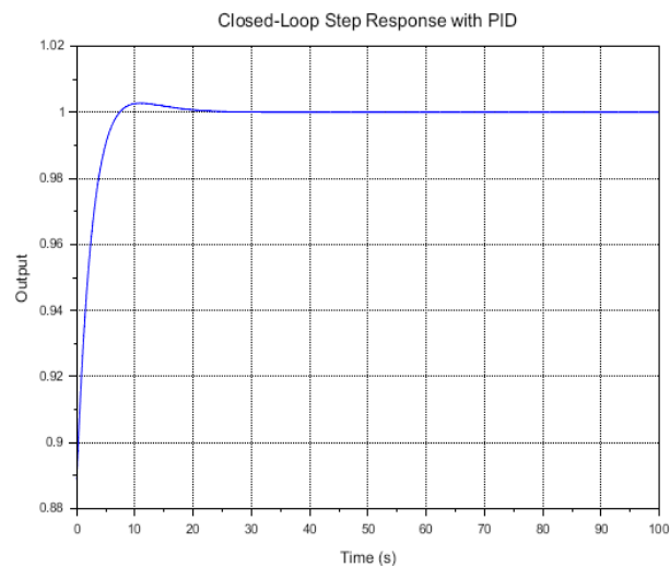
Gambar 17. Step Respon Kondisi Close Loop
