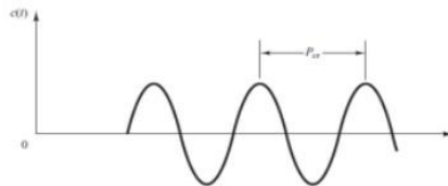
Gambar 11. Periode PCR dari Isolasi (Sumber : Hamid dkk., 2021)
