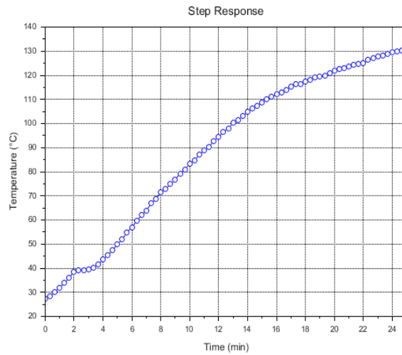
Gambar 16. Respon Sistem Kondisi Open Loop
