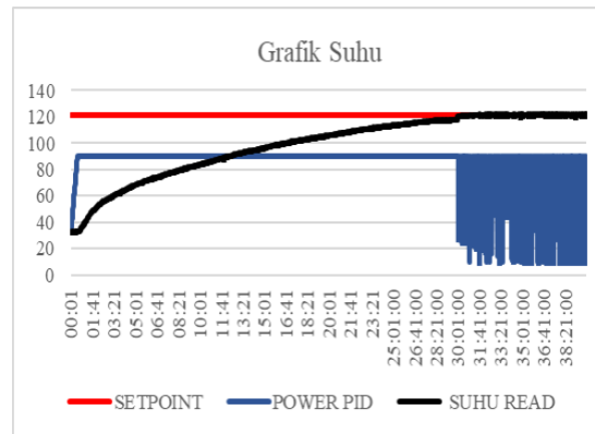
Gambar 19. Grafik suhu pada proses sterilisasi
